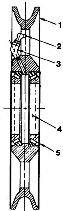
SECTION A-A
